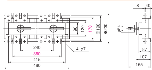
色:取付寸法 Mounting dimensions
