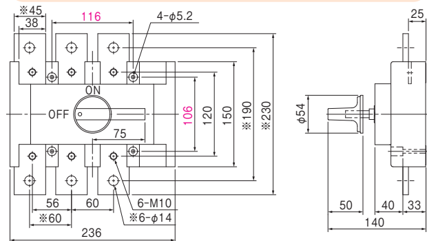
色:取付寸法 Mounting dimensions
