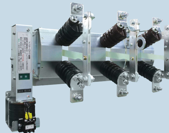
電氣的インターロック装置付き
