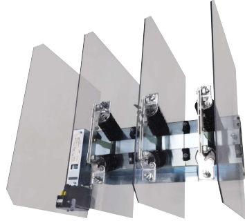
相間・アース間セパレータ (4枚) Interphase-Earth separators (4pcs.)
