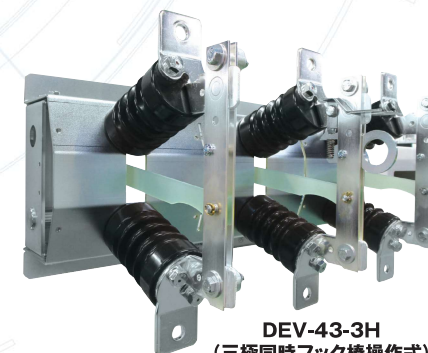
手動操作式(DD形)
