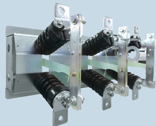
三極同時フック棒操作式
