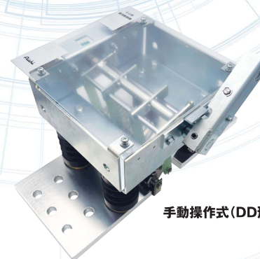
DEV-43-3E (電氣的インターロック装置付き)
